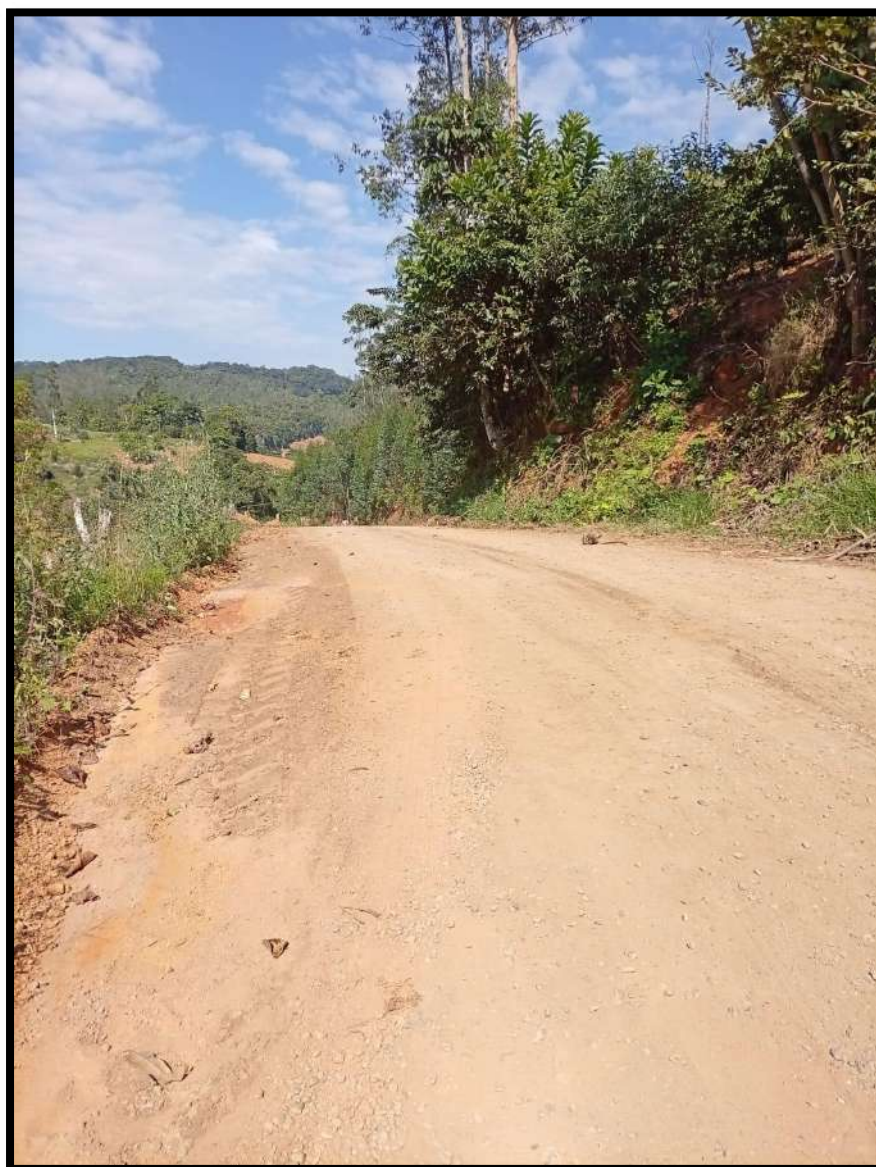
Fig. 03. Melhoramento do trecho com regularização da superfície utilizando motoniveladora.
